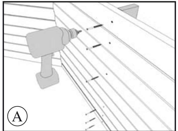
17e - Visser et noyer les têtes de vis.
