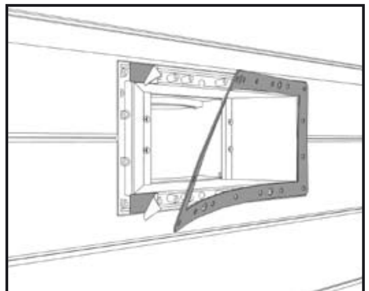
19e - Poser l'un des joints skimmer.
