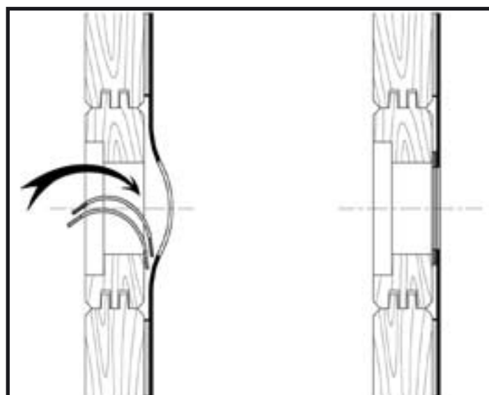
22e - Installer les joints de refoulement liège et caoutchouc.
