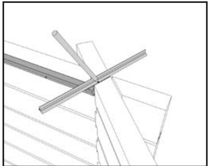
18d - Tracer l'angle à découper.
