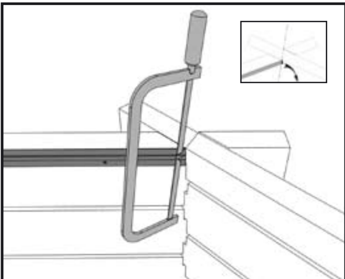
18e - Découper les angles selon le schéma.
