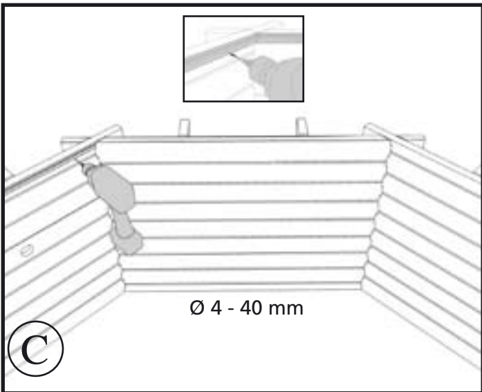
18c - Visser le premier rail du liner.
