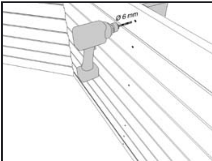
17d - Percer les parois.
