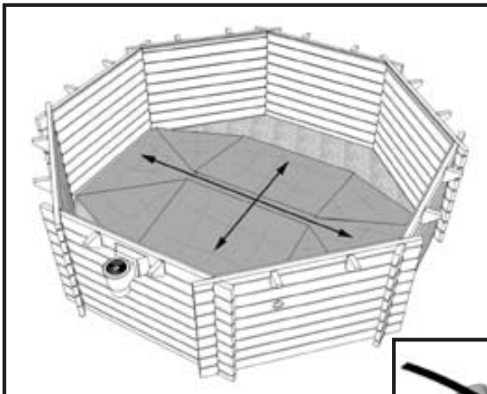
20d - Mettre en place le liner.
