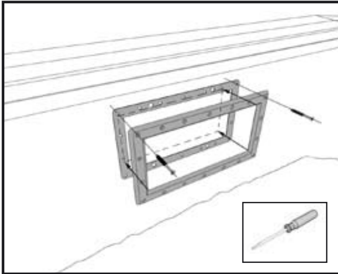
24c - Installer le joint et le cadre de skimmer.
