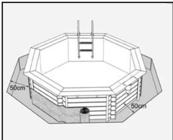
12b - Poser un film plastique isolant type DELTA MS (non fourni) sur la paroi extérieure pour drainer les eaux de pluie. La hauteur du film doit correspondre au niveau du remblai.
