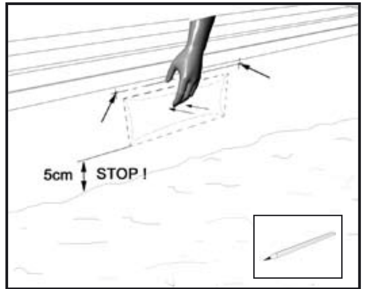
24b - Marquer l'emplacement du joint skimmer.
