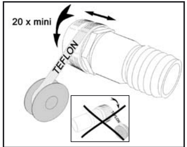
23b - Recouvrir la partie filetée des embouts à l'aide du ruban Téflon dans le sens anti-horaire. Minimum 20 tours.
