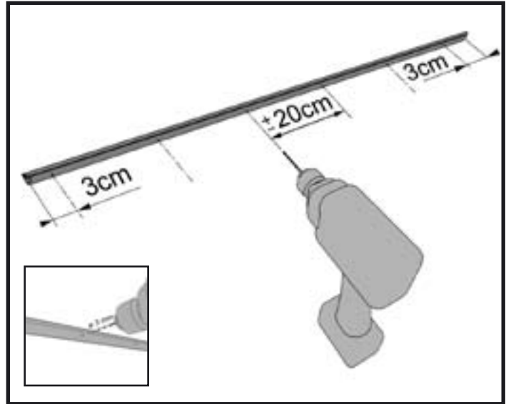
18b - Percer les rails aux dimensions (3 cm des extrémités puis tous les 20 cm environ).
