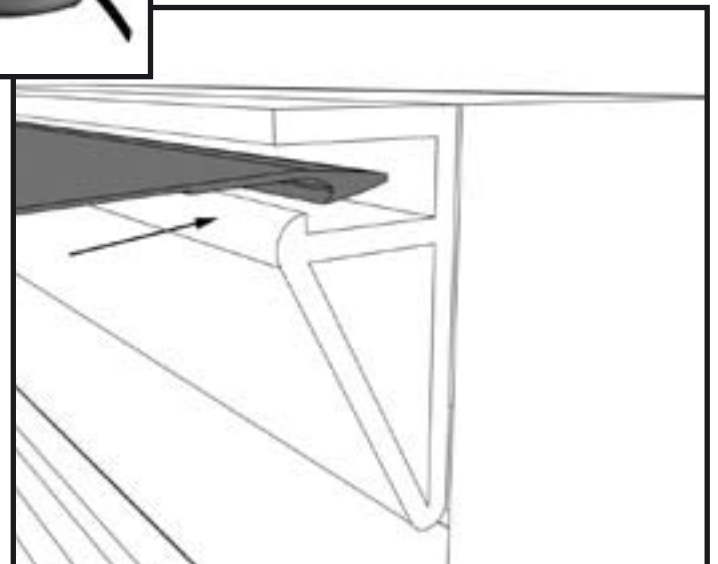
20e - Accrocher le liner dans la lèvre du rail.
