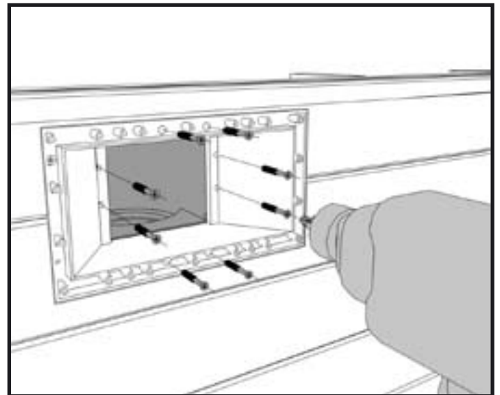
19c - Fixer l'ensemble en serrant efficacement pour une bonne étanchéité.
