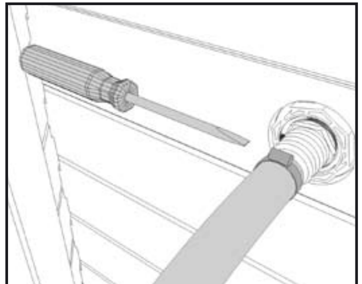
23c - Installer l'un des tuyaux de 4,50 m et le fixer à l'aide d'un collier métallique.
