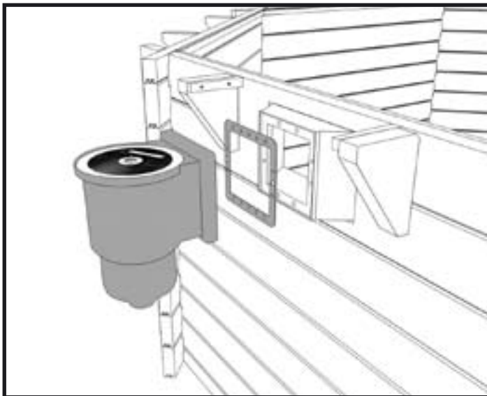
19b - Installer le joint extérieur skimmer ainsi que le corps du skimmer.
