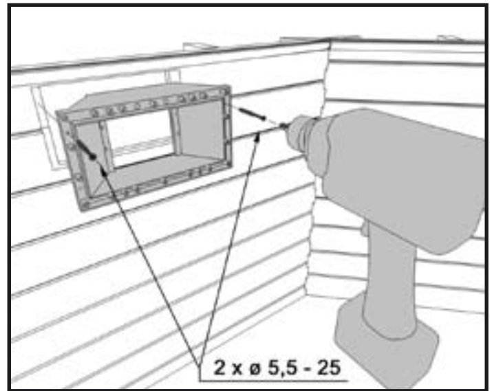
19a - Visser la bouche du skimmer dans le madrier supérieur à l'aide des vis fournies dans le carton du skimmer.
