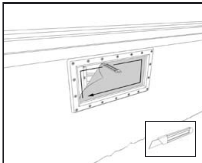
24d - Découper le liner à l'intérieur du cadre skimmer.
